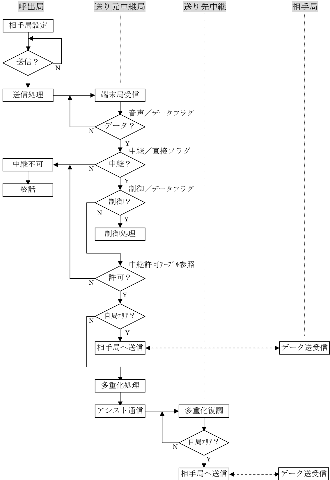
(1) 同一ゾーン内のデータ系通信フロー
