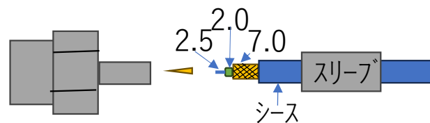
SMAコネクタ
