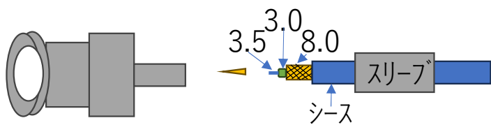
BNCコネクタ
